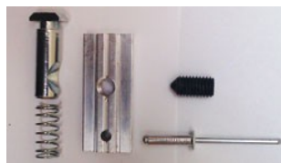
Zámok do stojky KOMBI / Lock for KOMBI upright
